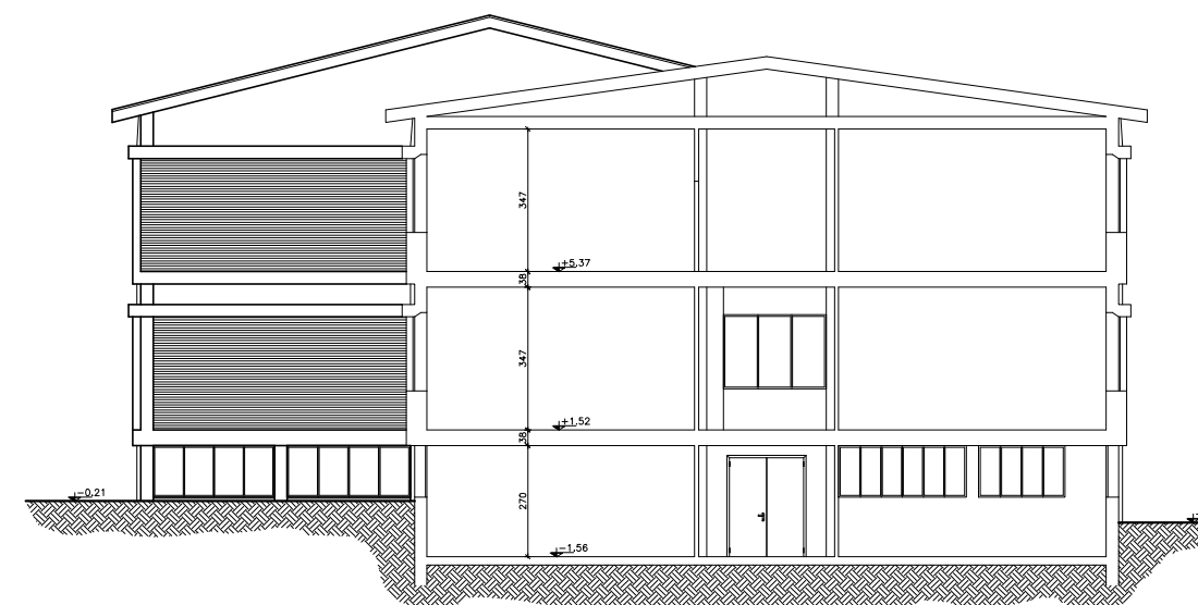
SEZIONE T-T
