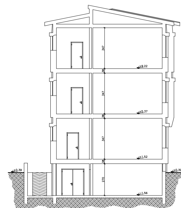
SEZIONE M-M
